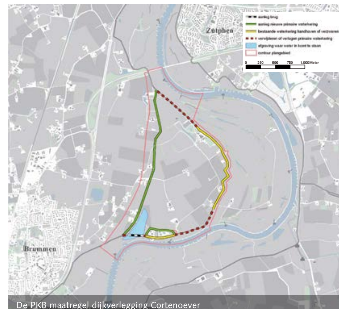
De PKB maatregel dijkverlegging Voorsterklei
