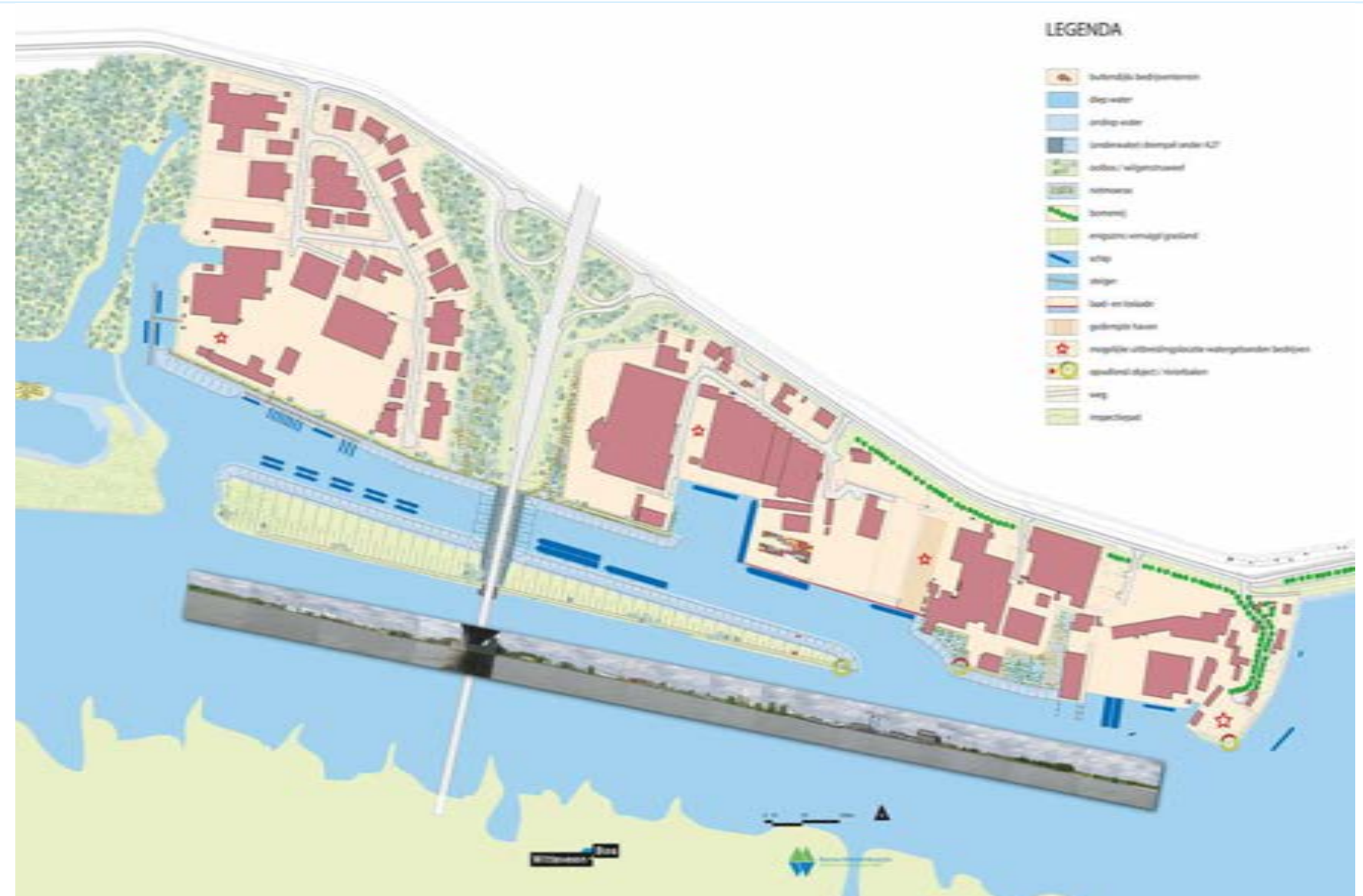
Inrichtingsplan
